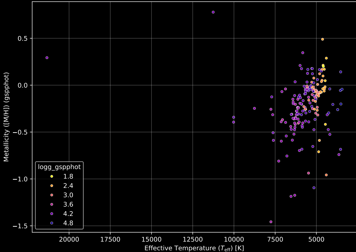
APOGEE DR17 Field: [CVZ_OB20_btx] Stellar Population Parameters (n= 185)
